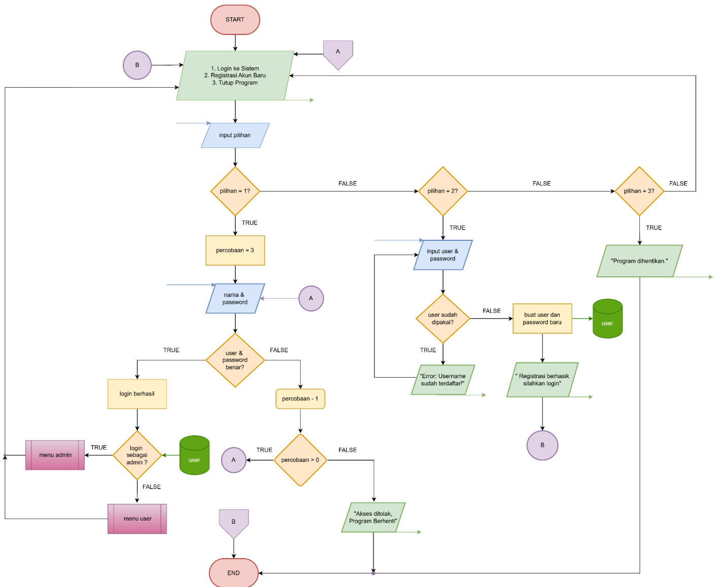
Gambar 2.1 Flowchart Utama
